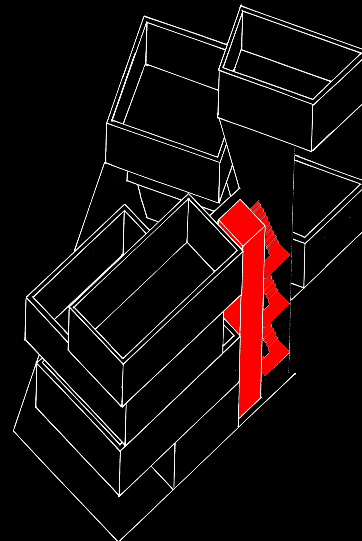
Axonometric 1:200
