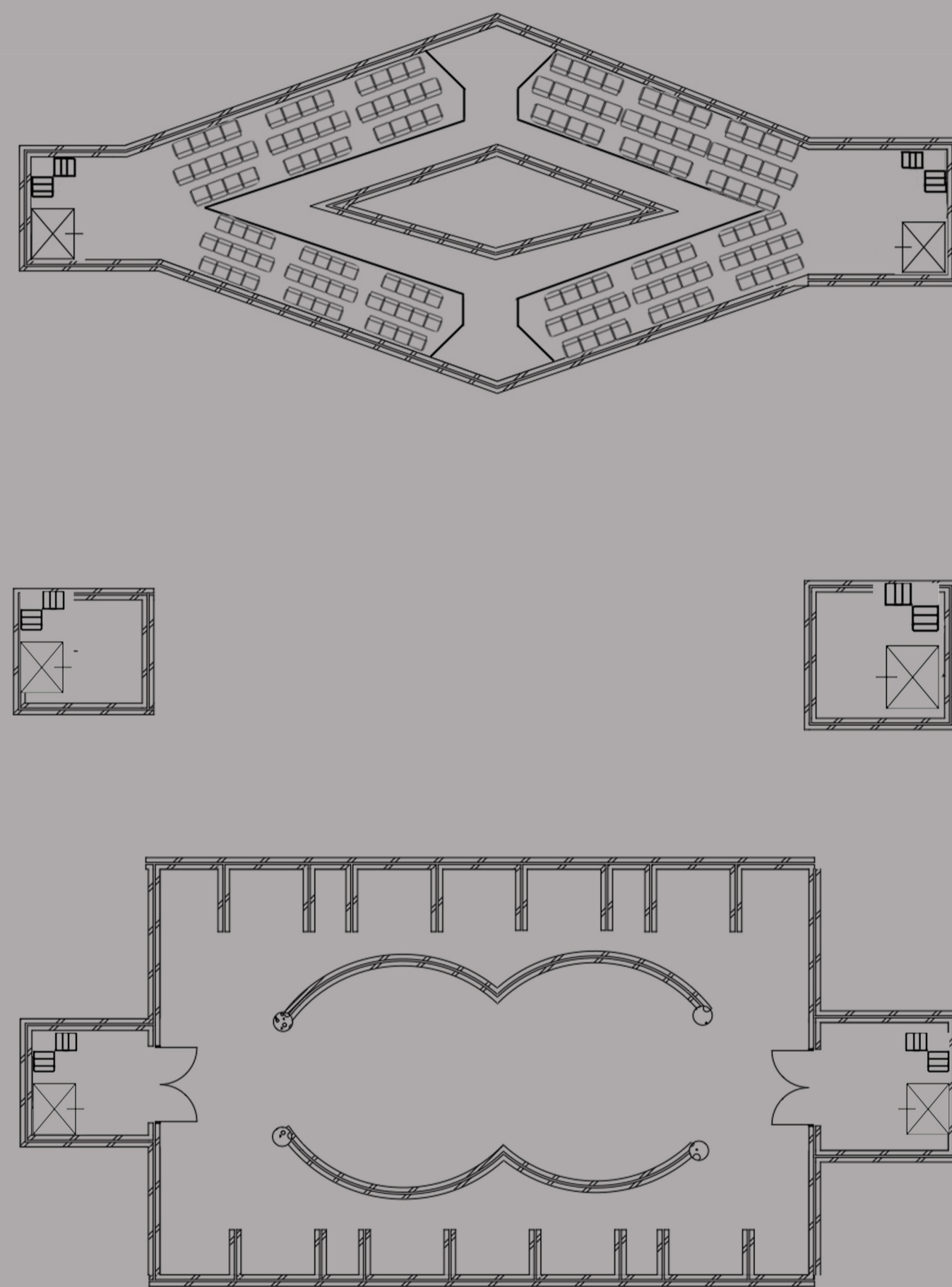
SITE PLAN 1:200
