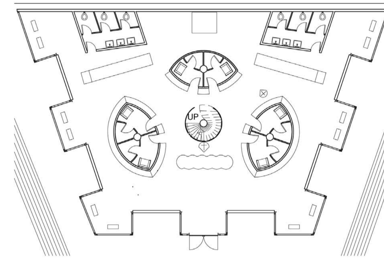
3 Level 1 1 : 200
