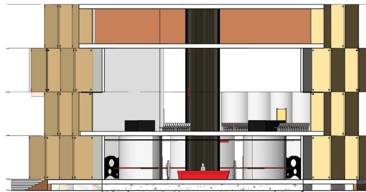
5 Section 1 1 : 200
