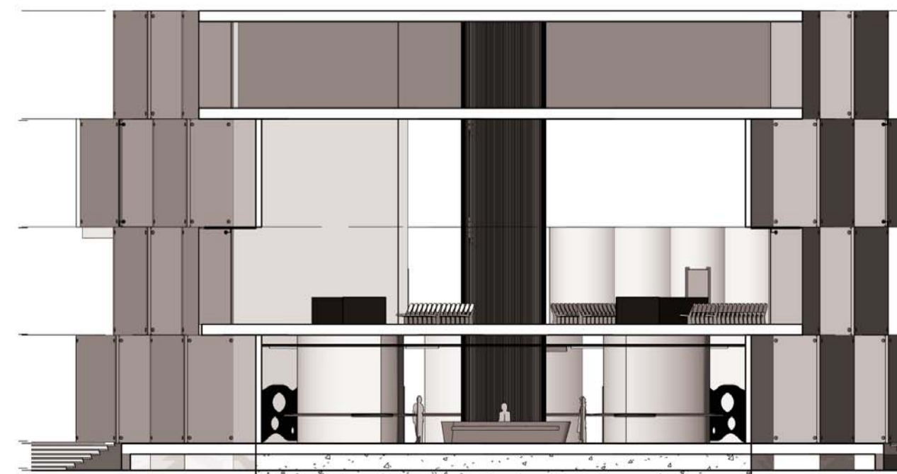
5 Section 1 1 : 200
