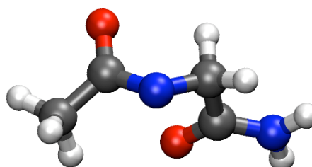
(b) \text{CH}_3\text{CO}\text{--}\bullet\text{N}\text{--}\text{CH}_2\text{CONH}_2
